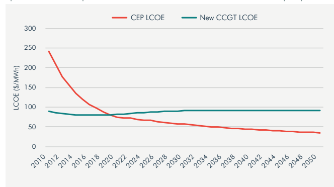
Figura 1. Confronto tra l'LCOE di un portafoglio di rinnovabili e quello di un impianto termoelettrico a ciclo combinato proposto
