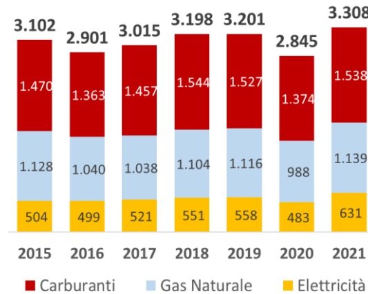
Figura 3 - Evoluzione spesa energetica annua della famiglia tipo
