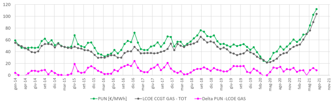
Figura 2 – Stretta correlazione tra PUN e costo di produzione energia elettrica da cicli combinati a gas (LCOE gas)
