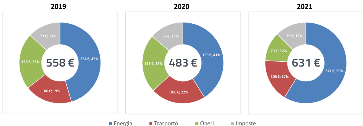
Figura 4 - Evoluzione della bolletta elettrica media annua della famiglia tipo e delle sue componenti (escluso canone TV)
